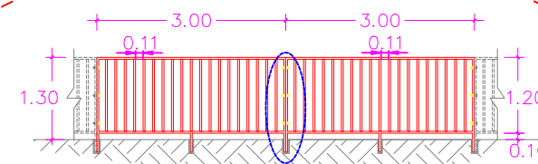
DETALHE GUARDA CORPO SEM ESCALA
